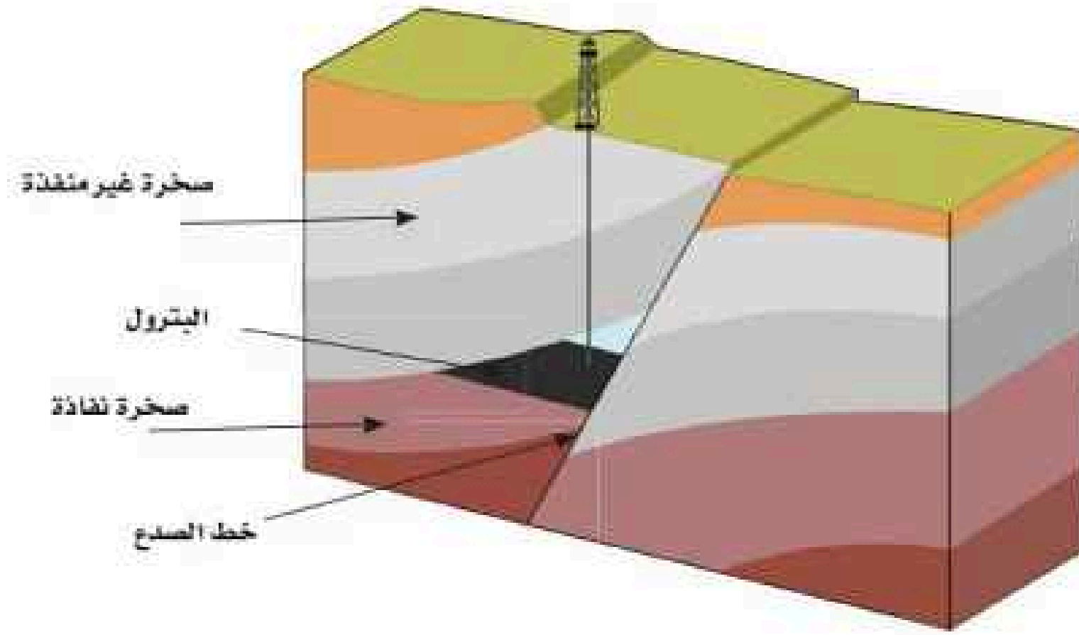
الشكل 4-5 مصادد الصدوع.
