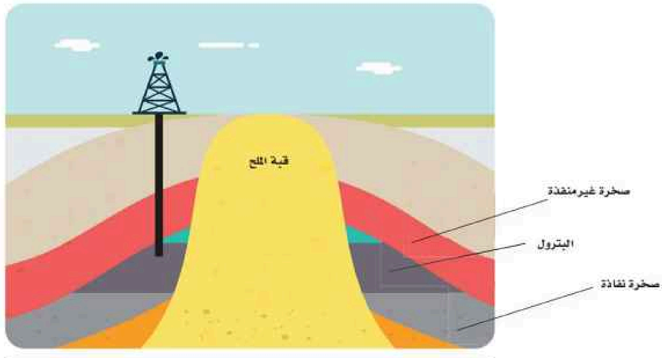
الشكل 5-5 مصادد القباب الملحية.
