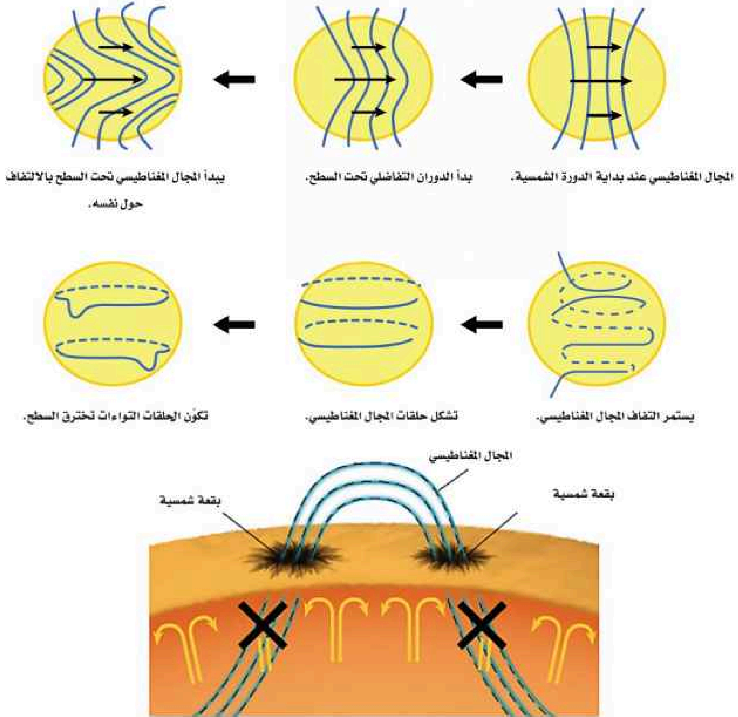
الشكل 2-7 التواء خطوط المجال المغناطيسي بسبب الدوران التفاضلي للشمس ونشوء البقع الشمسية.
