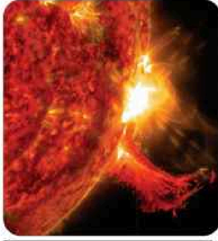
الشكل 9-2 التوهجات الشمسية.
