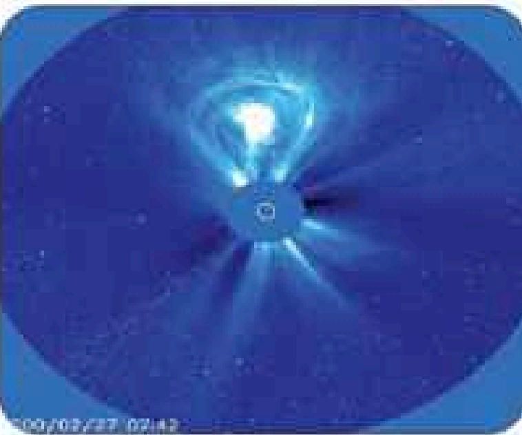
الشكل 11-2 الانبعاث الكتلي الإكليلي.
