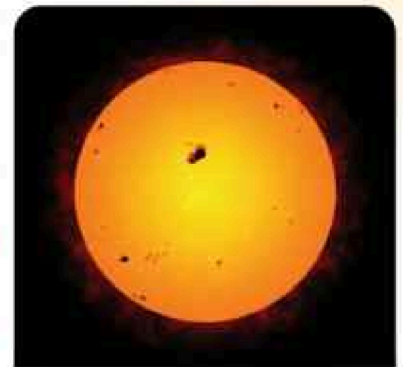
الشكل 2-8 البقع الشمسية على سطح الشمس.
