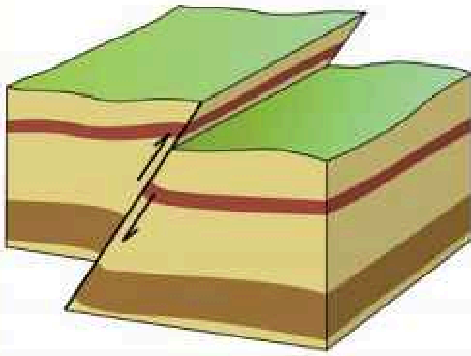
نموذج لمكمن صدعي.
