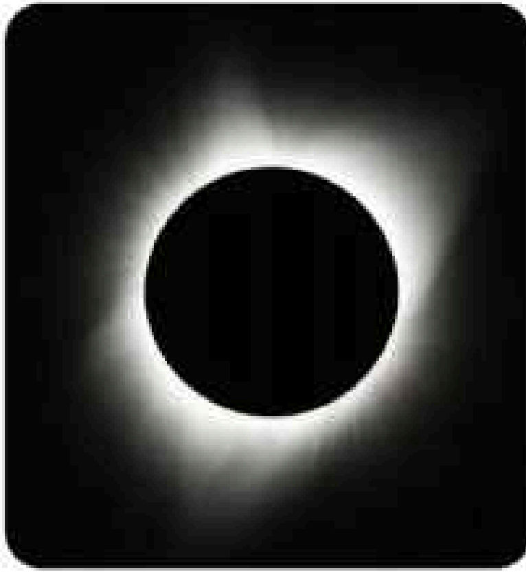
الشكل 2-6 طبقة الإكليل.
