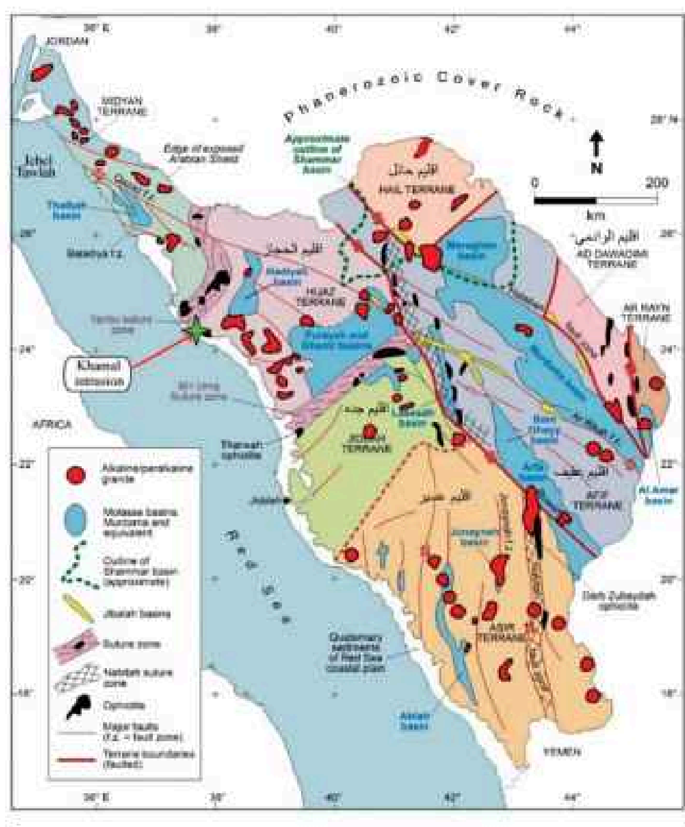
الشكل 3-6 خريطة توضح مواقع أقاليم الدرع العربي.
