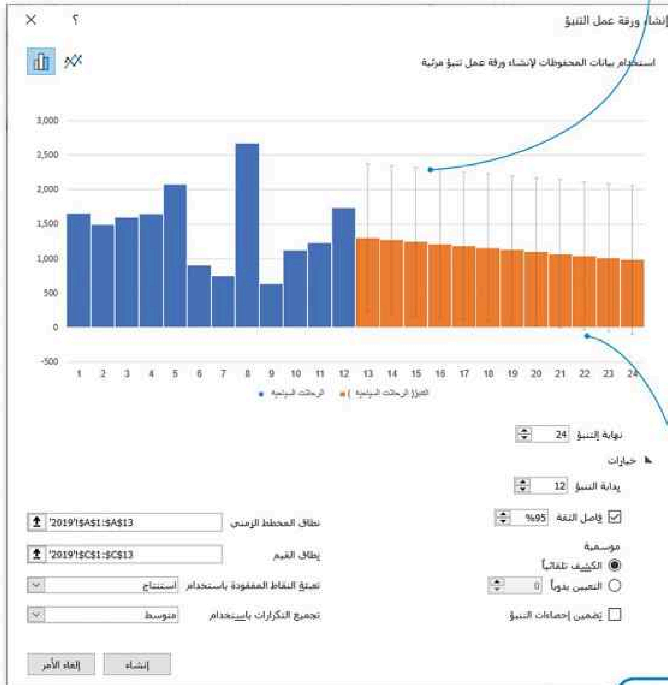
شكل 4.14: المخطط العمودي
