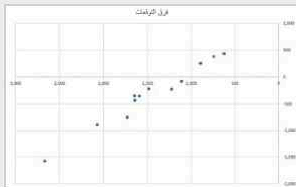
شكل 4.26: مخطط مبعثر
