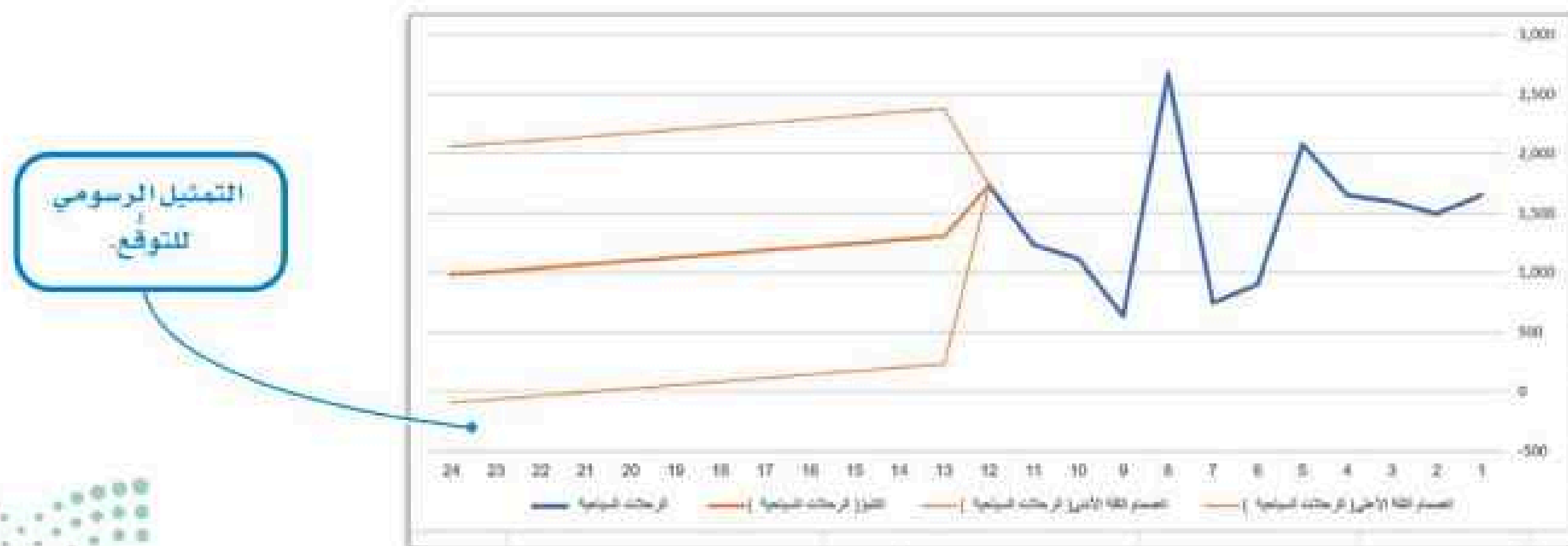
شكل 4.11: إنشاء التوقع
