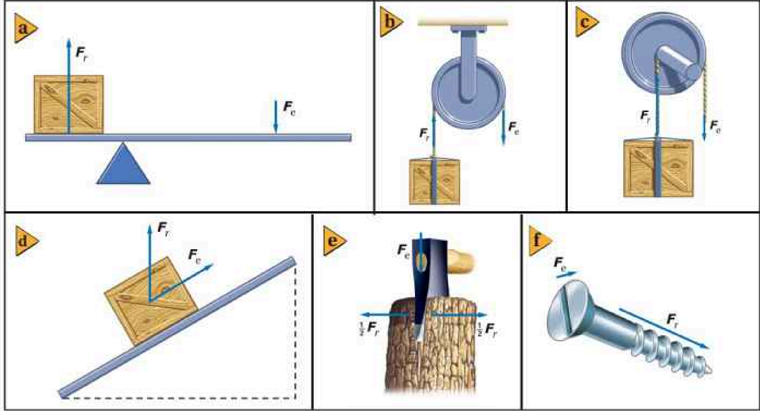
■ الشكل 11-4 آلات بسيطة تشتمل على (a) رافعة، (b) بكرة، (c) عجلة ومحور، (d) مستوى مائل، (e) إسفين (وتد) و (f) برغي.
