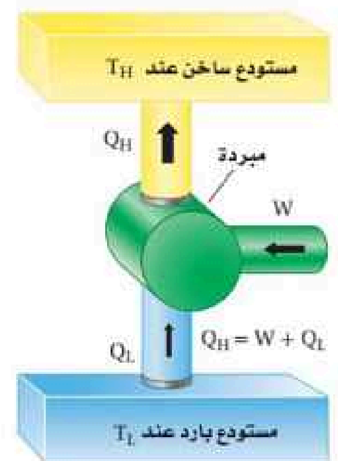
الشكل 6-13 يمتص المبرّد الحرارة Q_L من المستودع البارد ويبيعث الحرارة Q_H إلى المستودع الساخن، ببذل شغل W على المبرّد.
