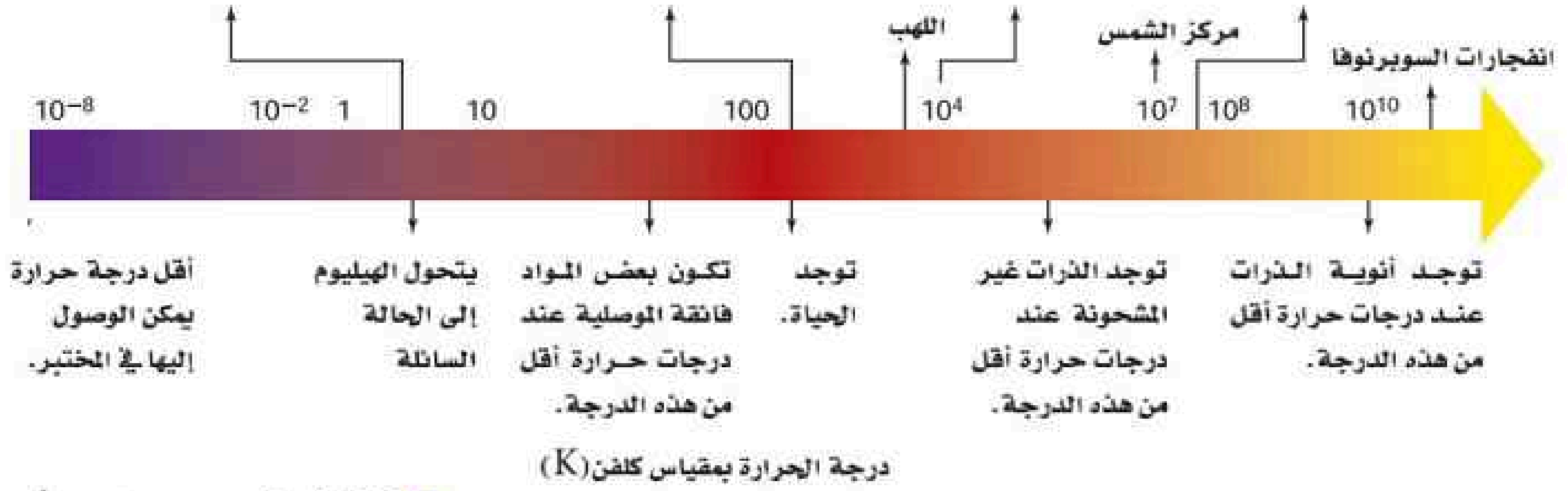
الفضاء (بين النجوم)
