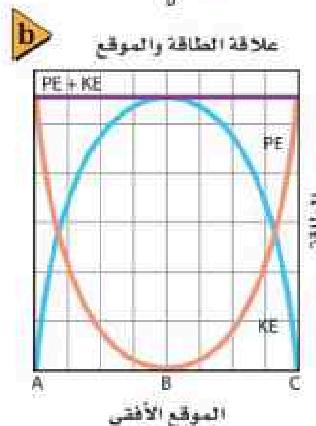
طاقة الوضع. طاقة الحركة. الطاقة الكلية للنظام في أي موقع تساوي مقدار ثابت.
