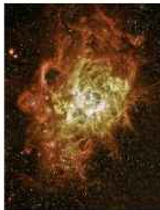
صورة هابل للمجرة NGC 6240
