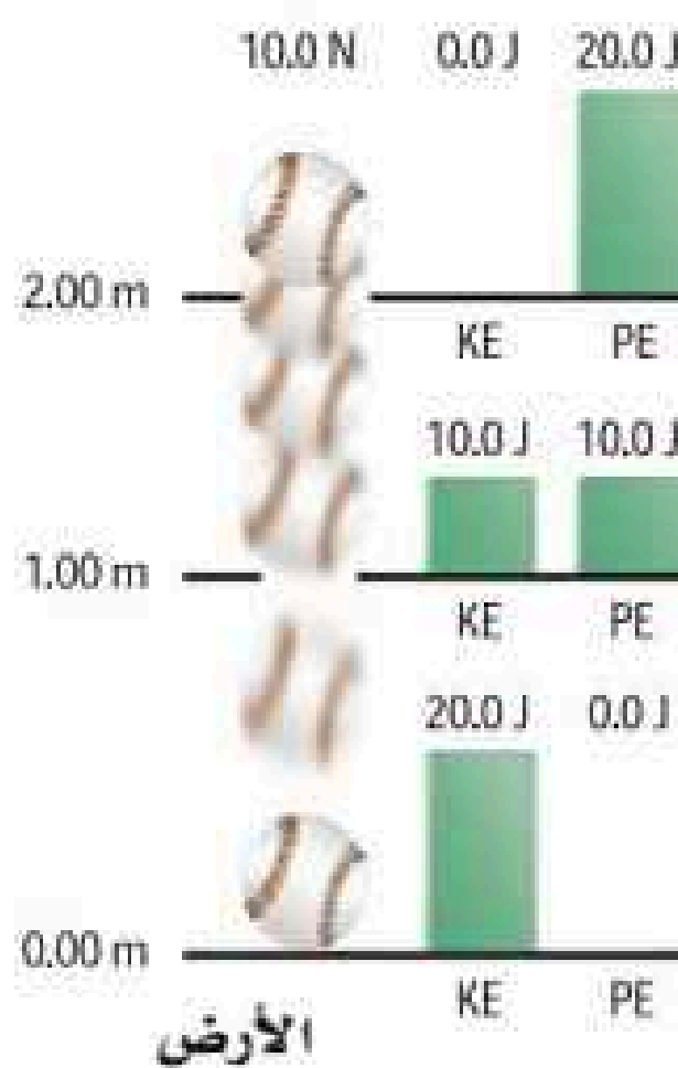
الشكل 5-9 انقصر في طاقة الوضع يساوي الزيادة في الطاقة الحركية.
