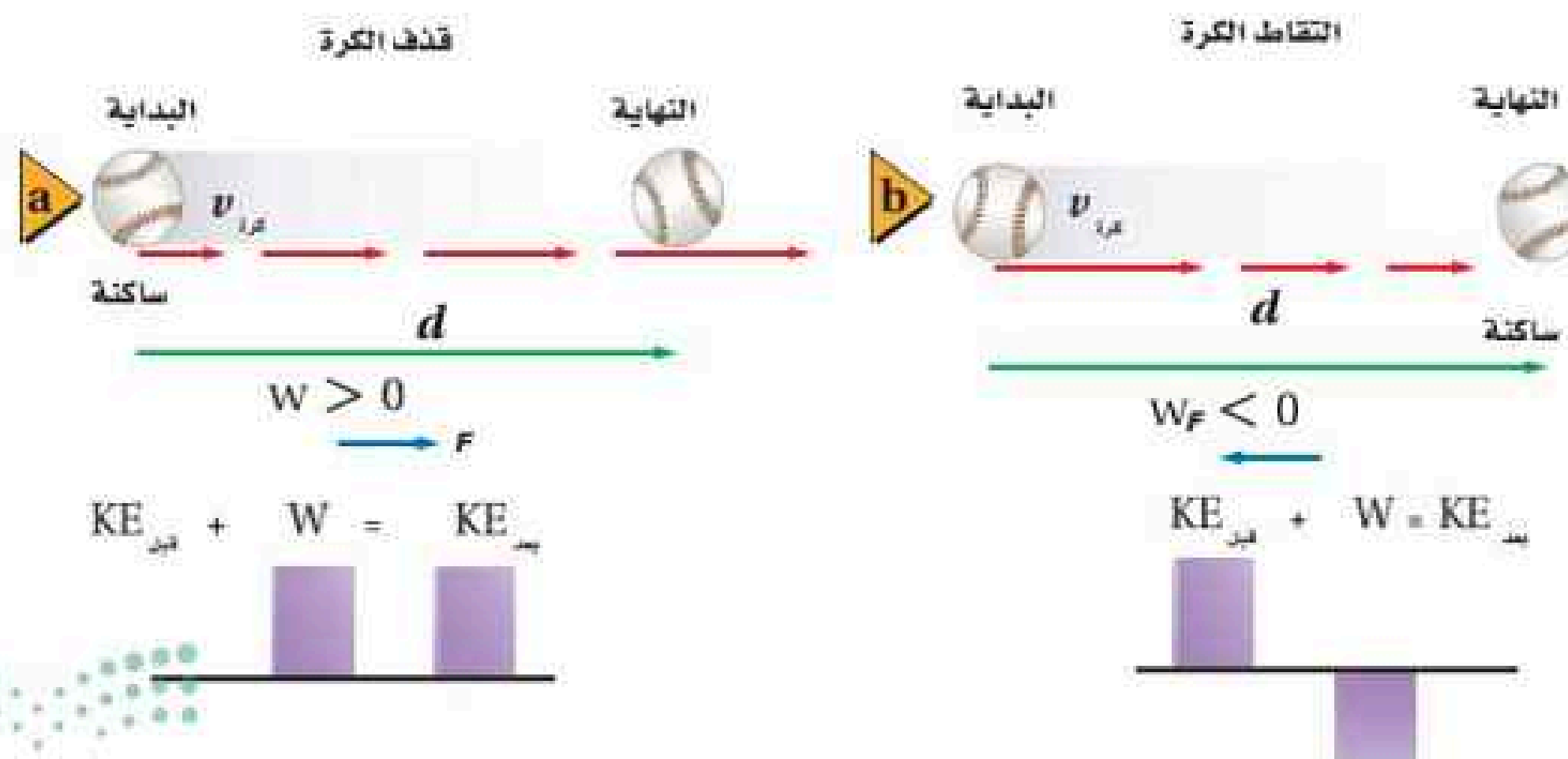
الشكل 5-2 الطاقة الحركية بعد قذف الكرة أو التقاطها تساوي الطاقة الحركية قبل عملية القذف أو الالتقاط + الشغل المبذول.
