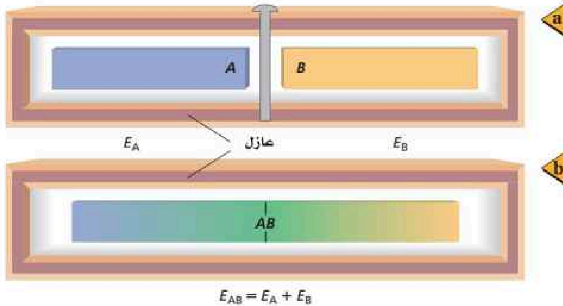
■ الشكل 6-8 نظام مكون من نموذجين لثلاثين عند درجات حرارة مختلفة، وهما مفصولان في الحالة الابتدائية (a). وعندما يتلامس الثالبان فإن الحرارة تتدفق من الثالب الساخن إلى الثالب الأبرد (b). وتبقى الطاقة الكلية ثابتة.
