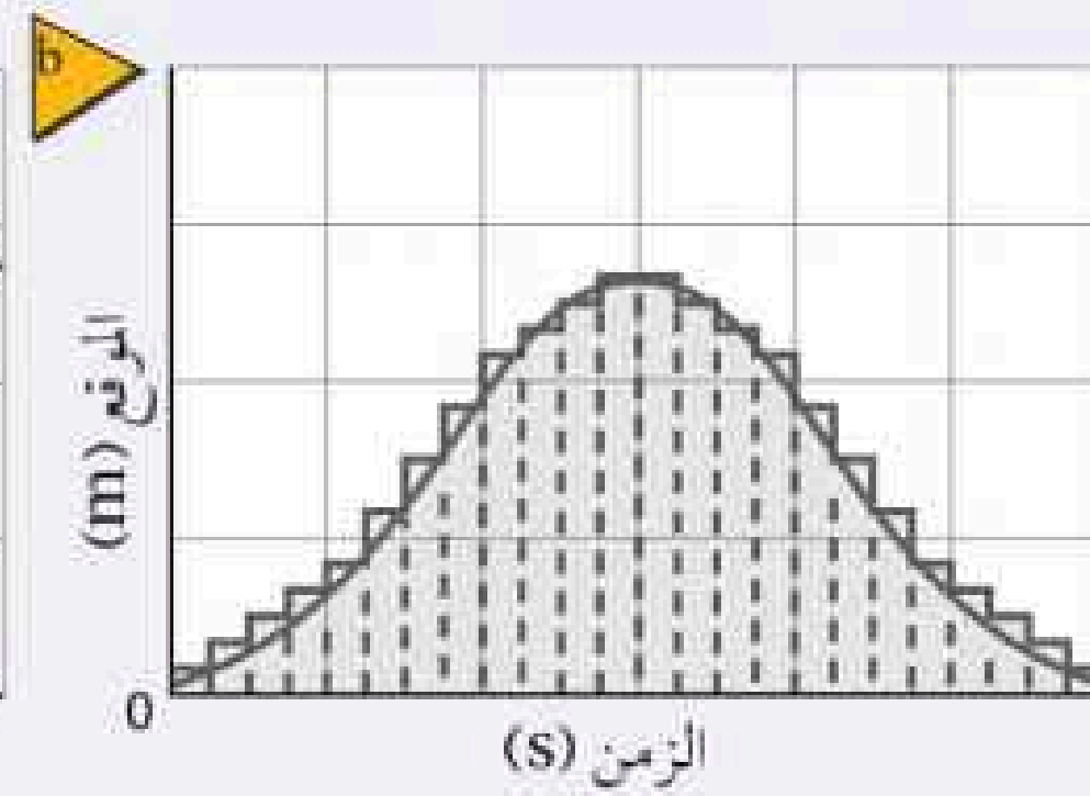
المساحة الإجمالية تساوي المساحة 1 + المساحة 2 + المساحة 3 + ...
