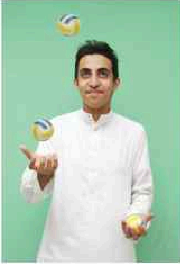
■ الشكل 5-5 تتغير طاقة وضع الكرة وطاقتها الحركية باستمرار عند قذفها إلى أعلى كما يفعل اللاعب.
