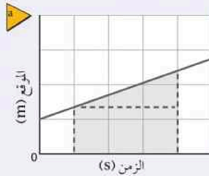
المساحة الإجمالية تساوي مساحة المستطيل + مساحة المثلث
