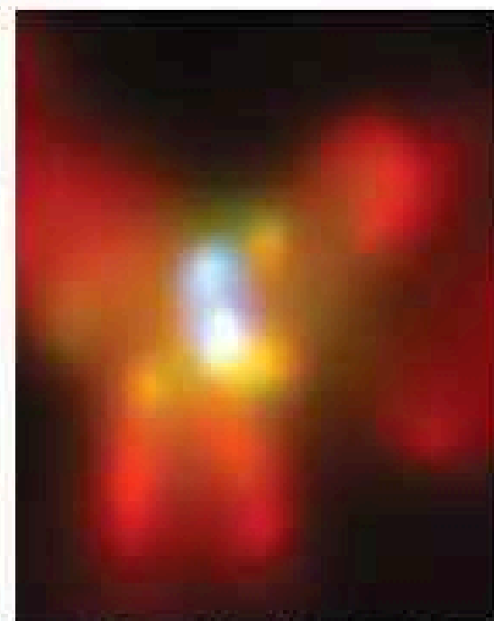
صورة شادرا بالأشعة السينية لتقنين أسودين في NGC 6240
