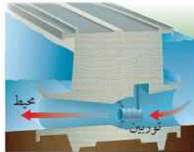
أ خلال الجزر، تفتح البوابة ويتدفق الماء من السد عبر التوربين فيدير المولد الكهربائي من جديد.
