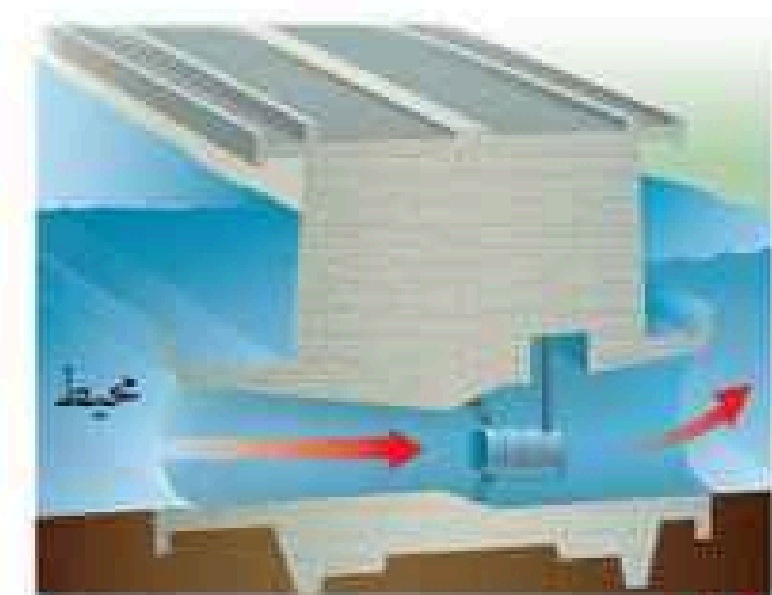
ب خلال المد تدبر حركة الماء التوربين المرتبط مع المولد الكهربائي، وعند اكتمال المد تغلق البوابة لتحتجز الماء خلف السد.
