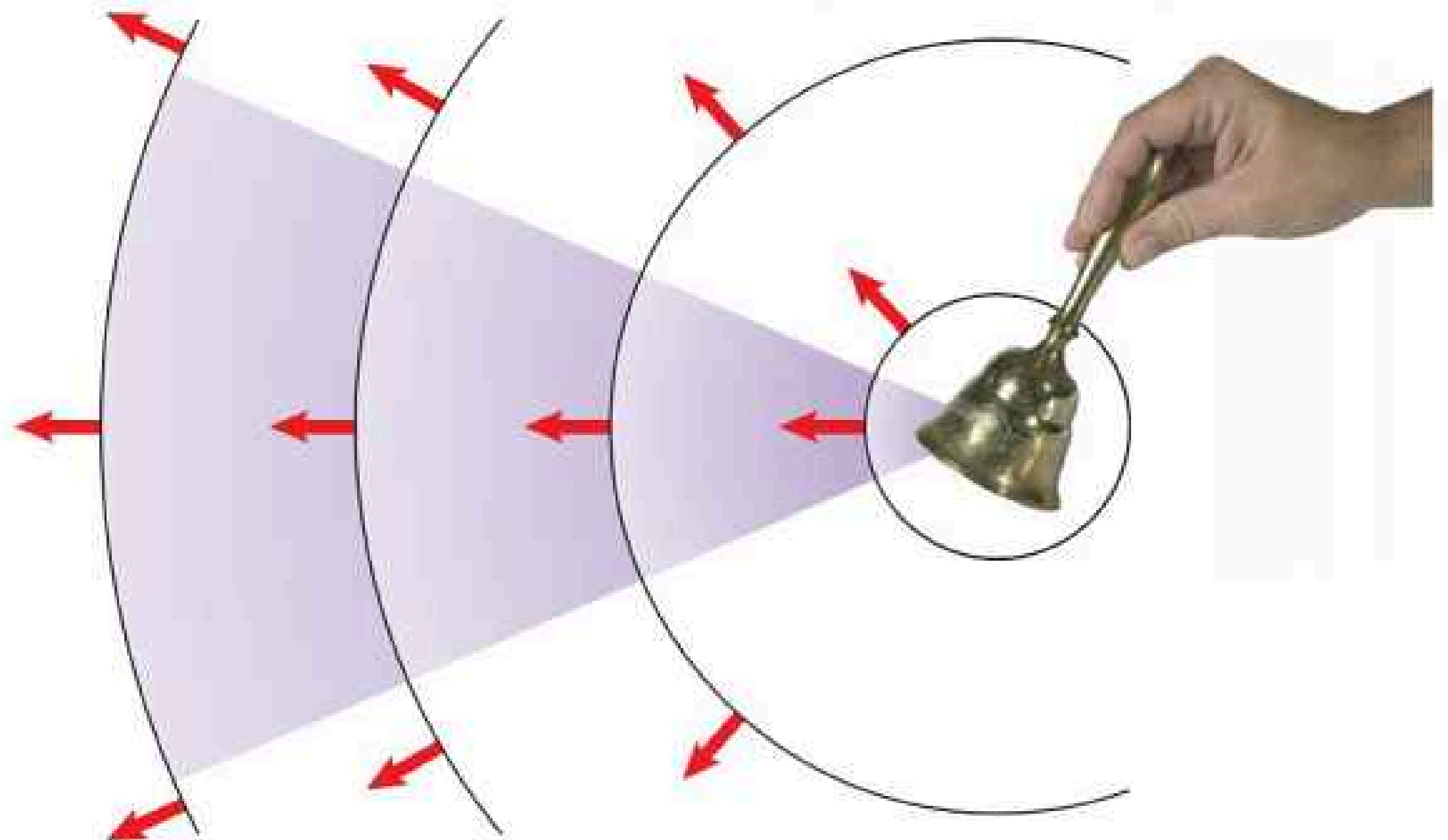
الشكل ١٢ تتناقص شدة موجات الصوت كلما انتشر الصوت مبتعداً عن مصدره؛ حيث تتوزع الطاقة التي تحملها موجات الصوت على مساحة أكبر.
