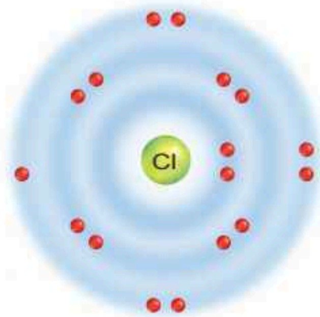
ذرة كلور
