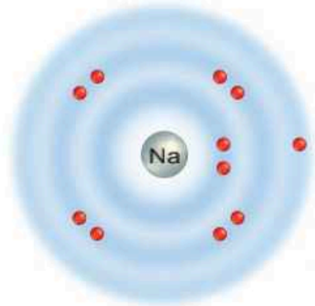
ذرة صوديوم
