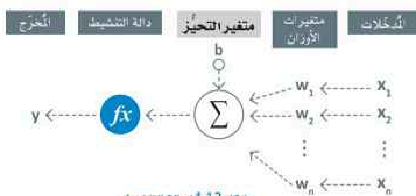
شكل 4.12: دالة التنشيط
