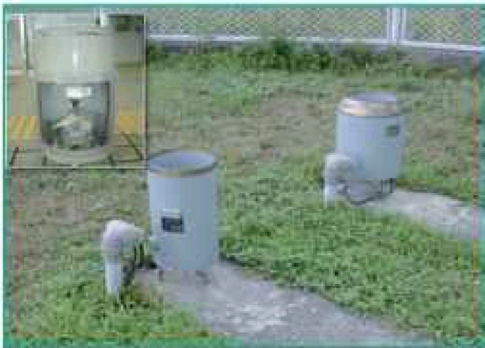
مقياس المطر
