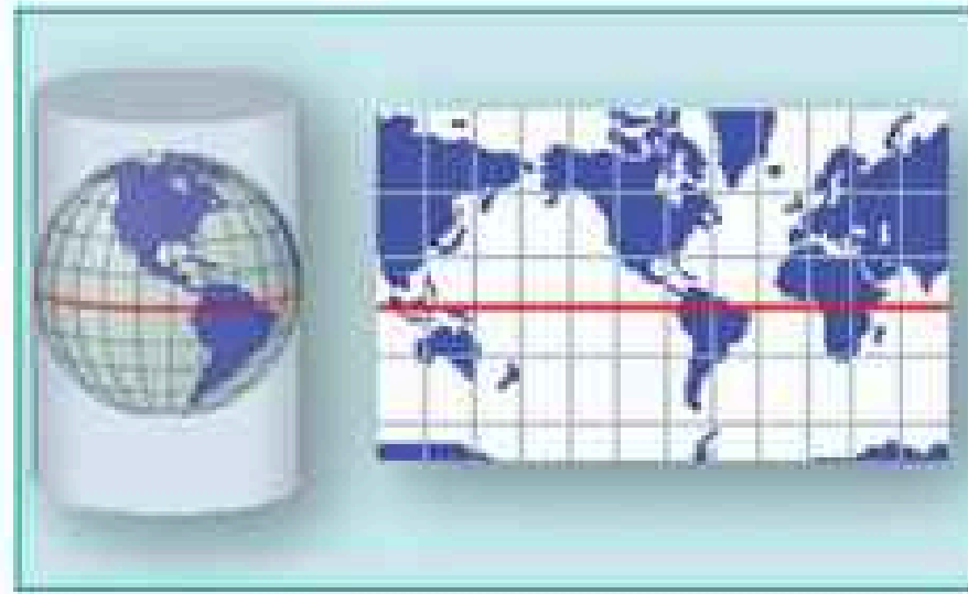
المسقط الأسطواني
