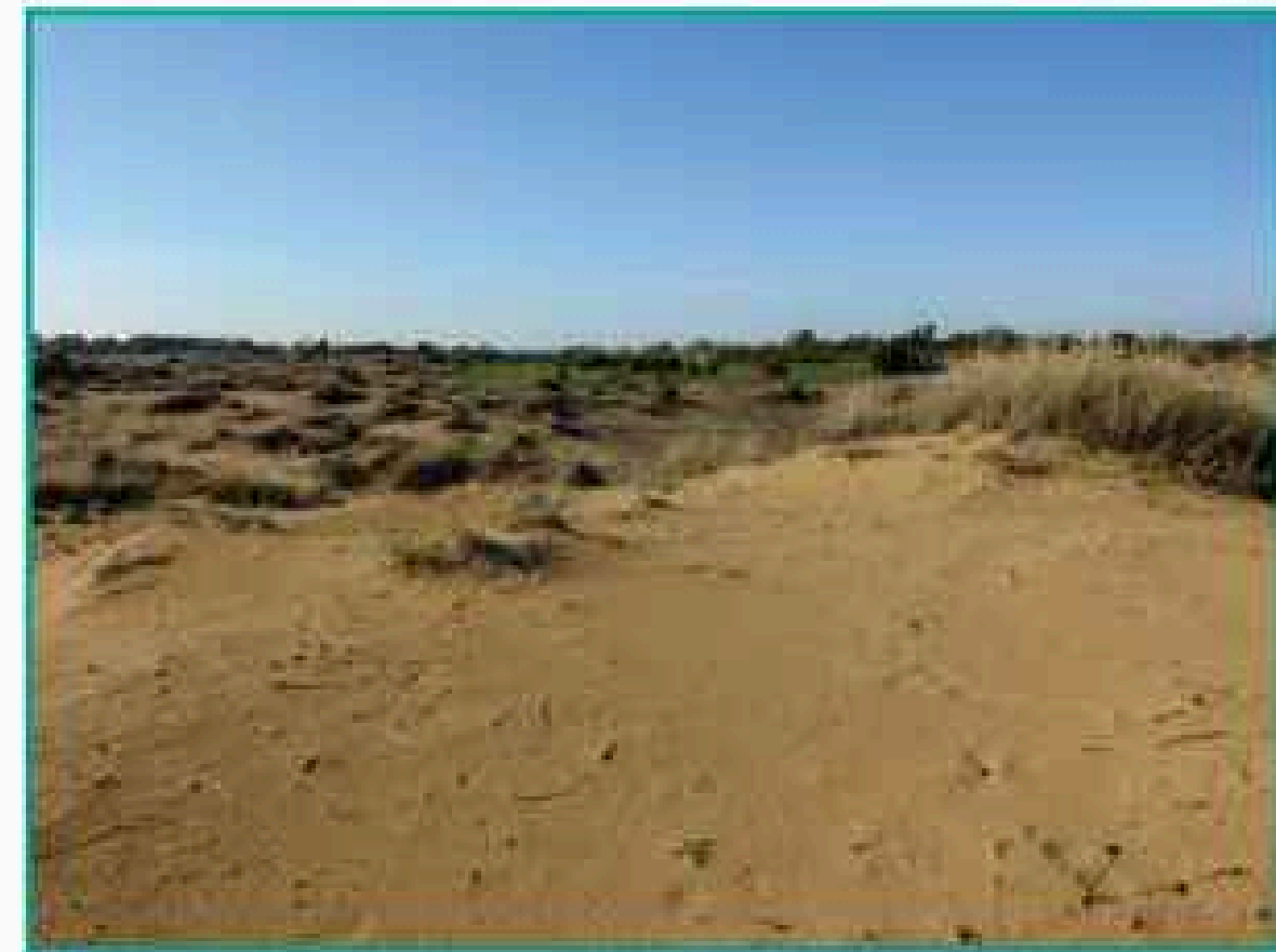
التصحّر
