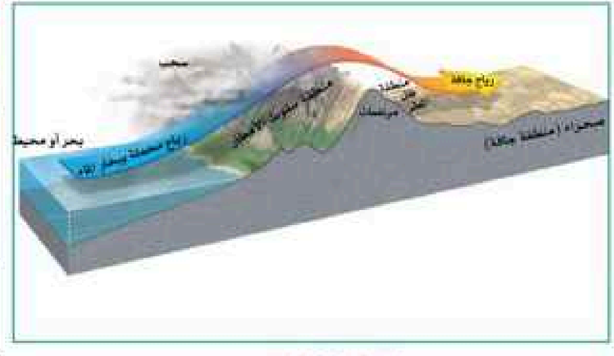
المطر التضاريسي
