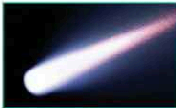
مذنب
