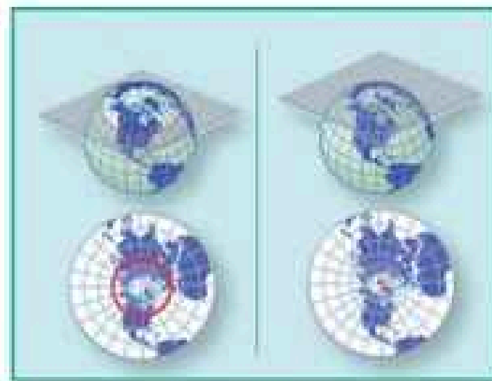
المسقط المستوي
