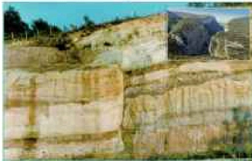
من أنواع الانكسارات
