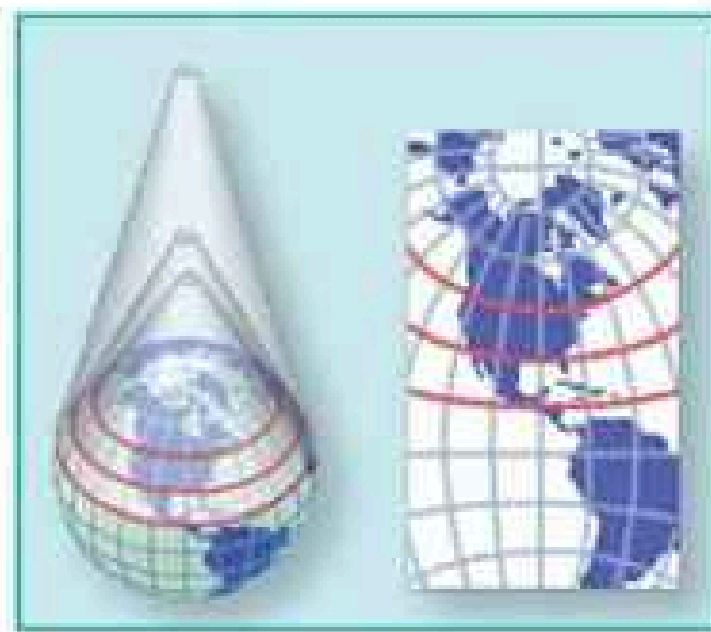
المسقط المخروطي
