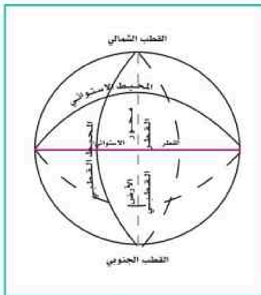
أبعاد الأرض
