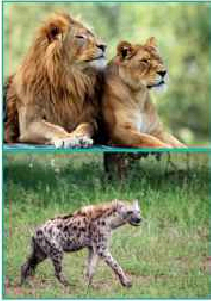
حيوانات مفترسة
